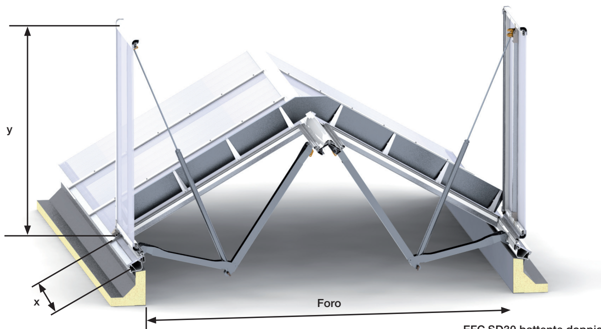
EFC SD30 battente doppio Esempio 250/100
