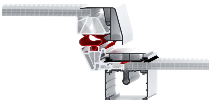
Schwallwasserlippe und integrierte Ballondichtung
