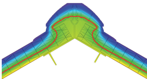
Profilo di colmo
