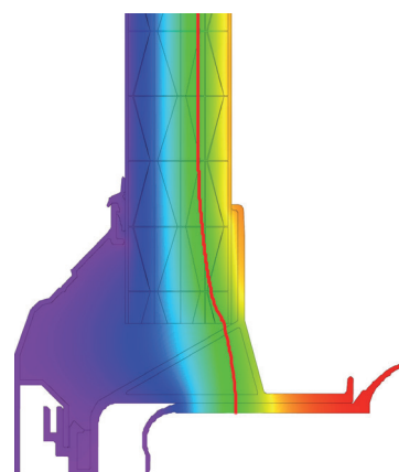
Profilo di base elemento frontale
