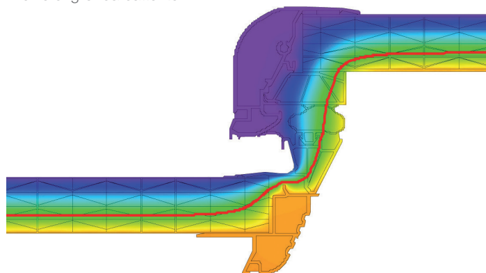
Profilo di gronda battente
