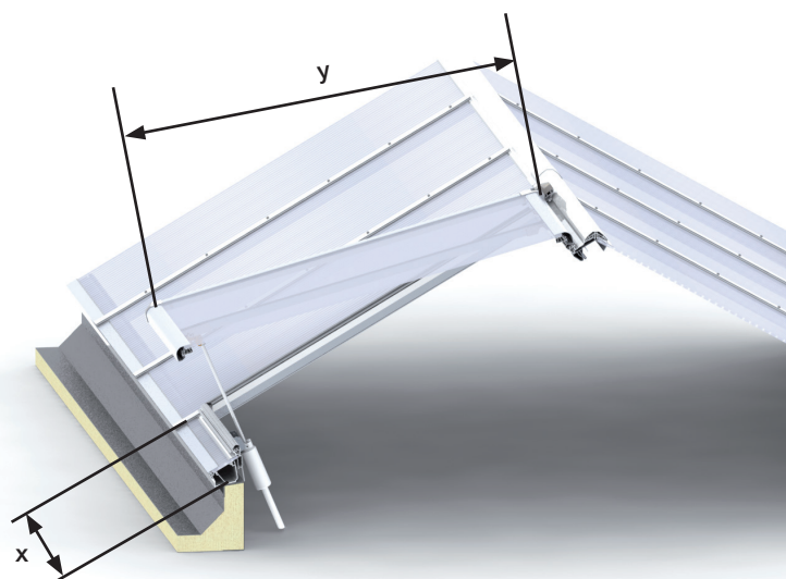
battente d'aerazione singolo
